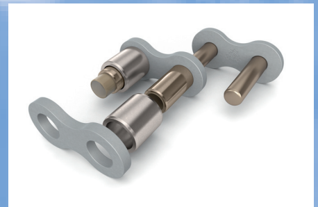
TRIATHLON KS Korrosionsbeständig und schmierstofffrei für hoch sensible Produktionsabläufe.
