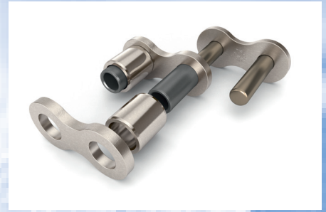
MARATHON Die Langlaufkette ohne Nachschmierung.
